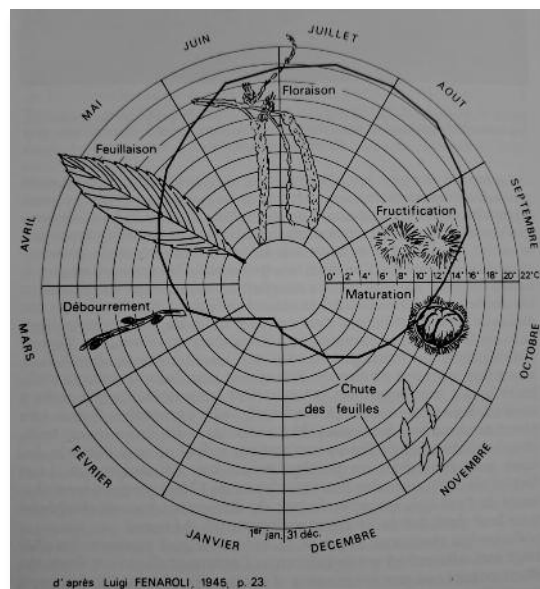
Cycle végétatif du châtaignier au regard des températures idéales moyennes.
